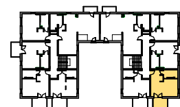
PLAN BUDYNKU
